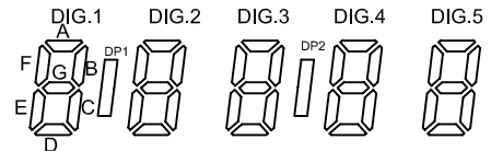
屏贴显示图
